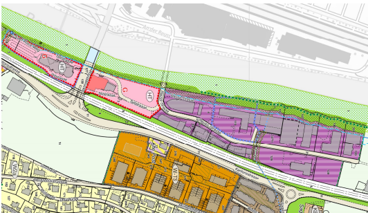
Abb. 16: Zonenplan neu: Arbeitszone AIII, Hotel- und Tourismuszone Tell
